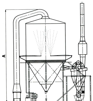
Essiccatoio a spruzzo con ugelli a pressione in versione con distribuzione assiale dell'aria calda.
