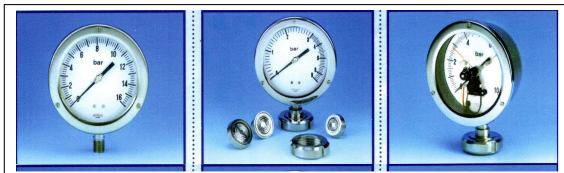
Manomètre acier inox Diam 130 – 150 0 à 400 bar
