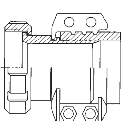
Système Coquille récupérable Reusable Ferrule system
